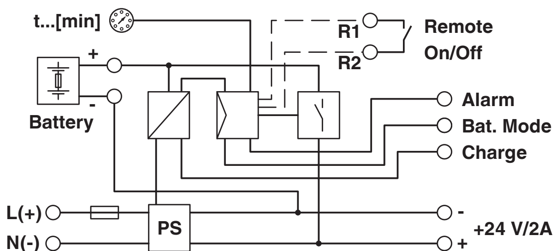
Blockschaltbild
