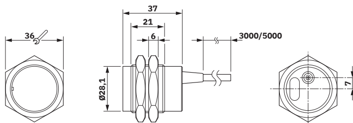
Esquema de dimensiones
