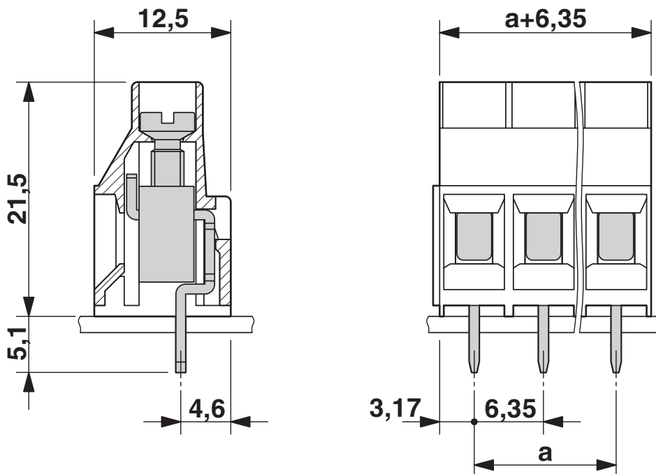
Maßzeichnung
