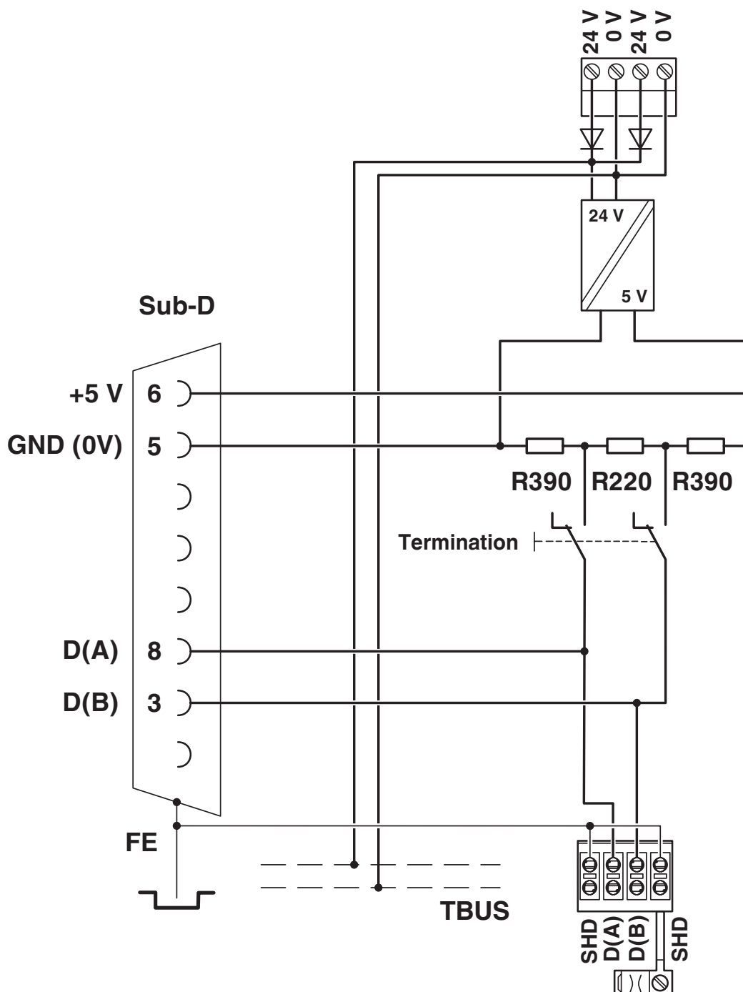
Schéma fonctionnel
