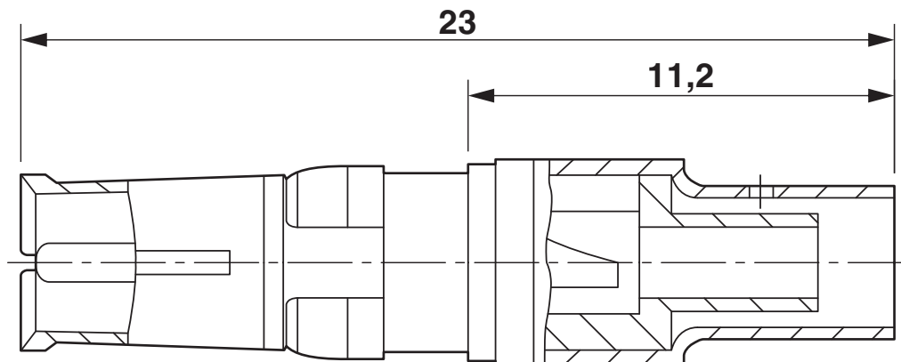
Contacto coaxial macho D-SUB
