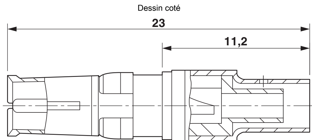
Contact coaxial mâle SUB-D
