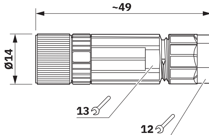
Maßzeichnung
