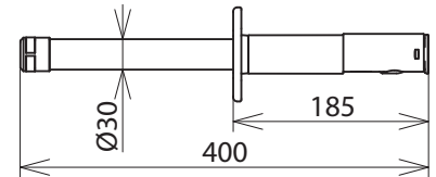
Maßbild EG SK STK 400
