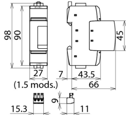
Dimensiones del DG SE DC 900 FM
