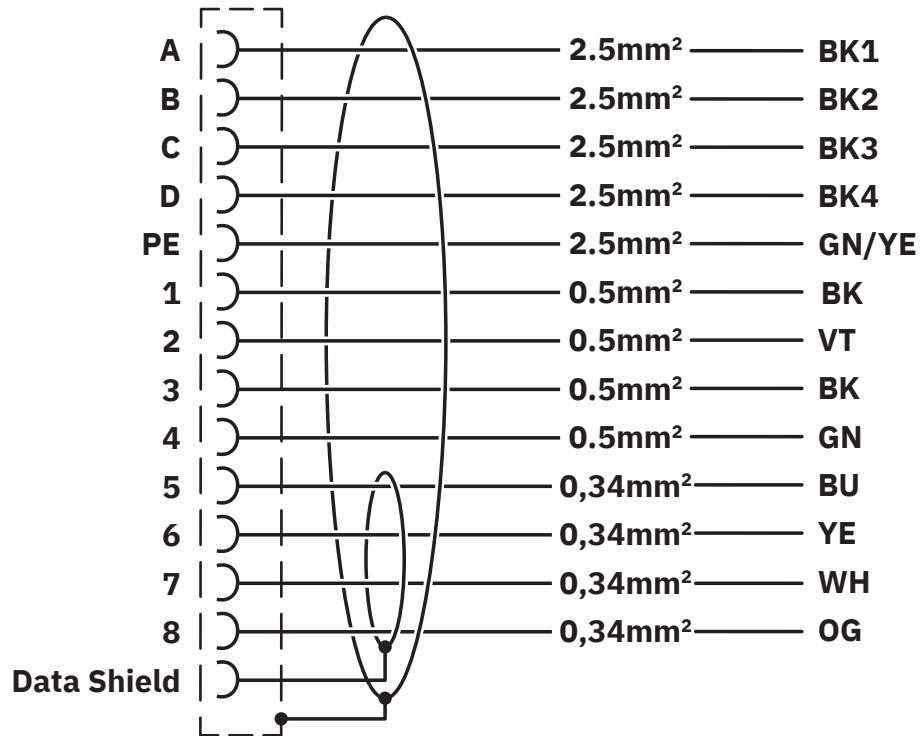
Diagrama eléctrico
