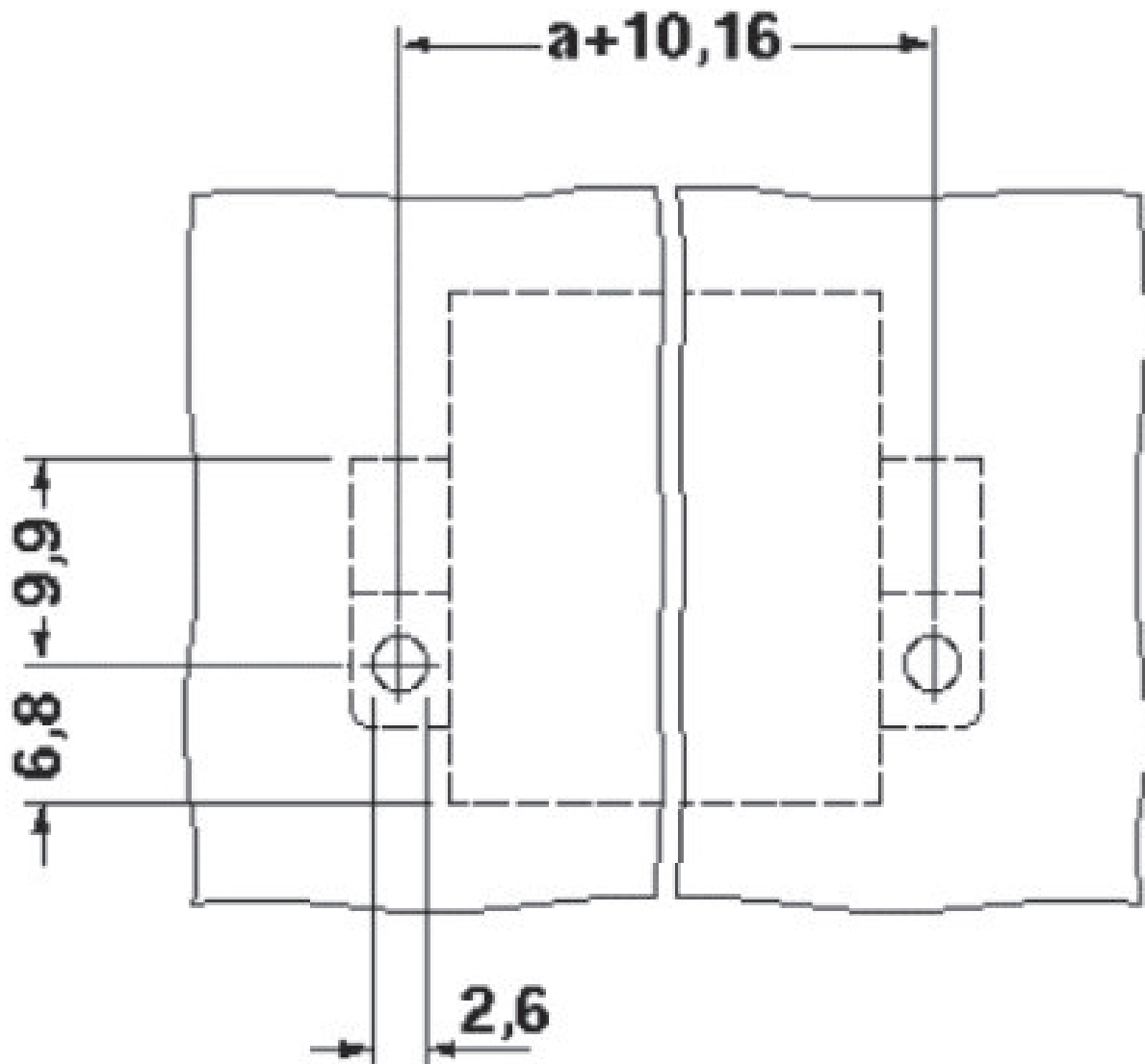
Bohrplan/Lötpadgeometrie
