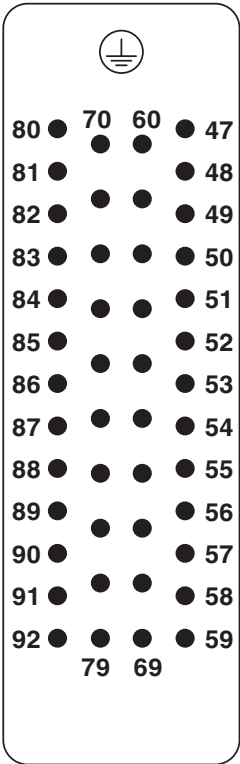
Plano esquemático
