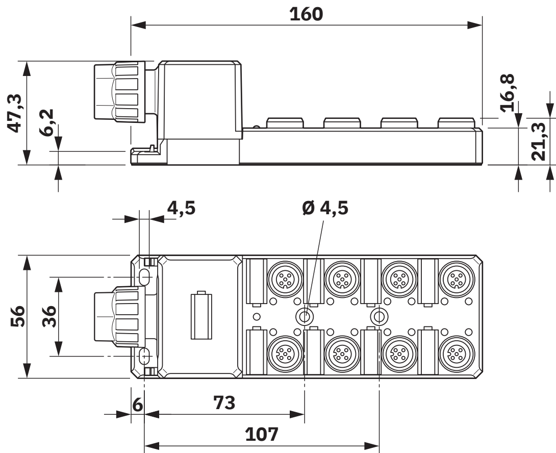
Dessin coté
