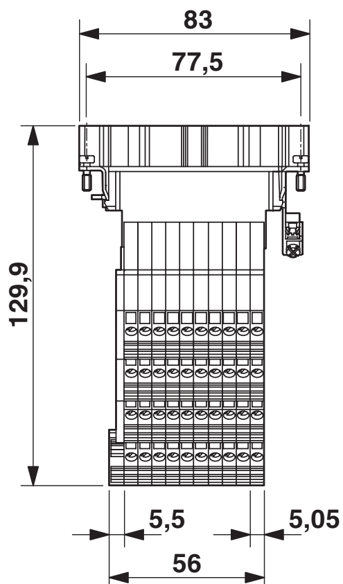
Esquema de dimensiones
