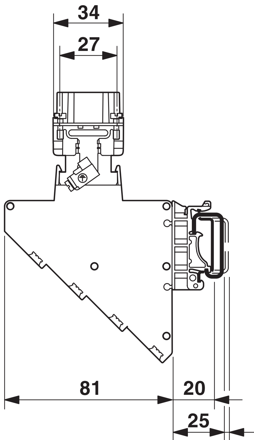
Dessin coté
