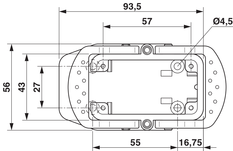
Maßzeichnung
