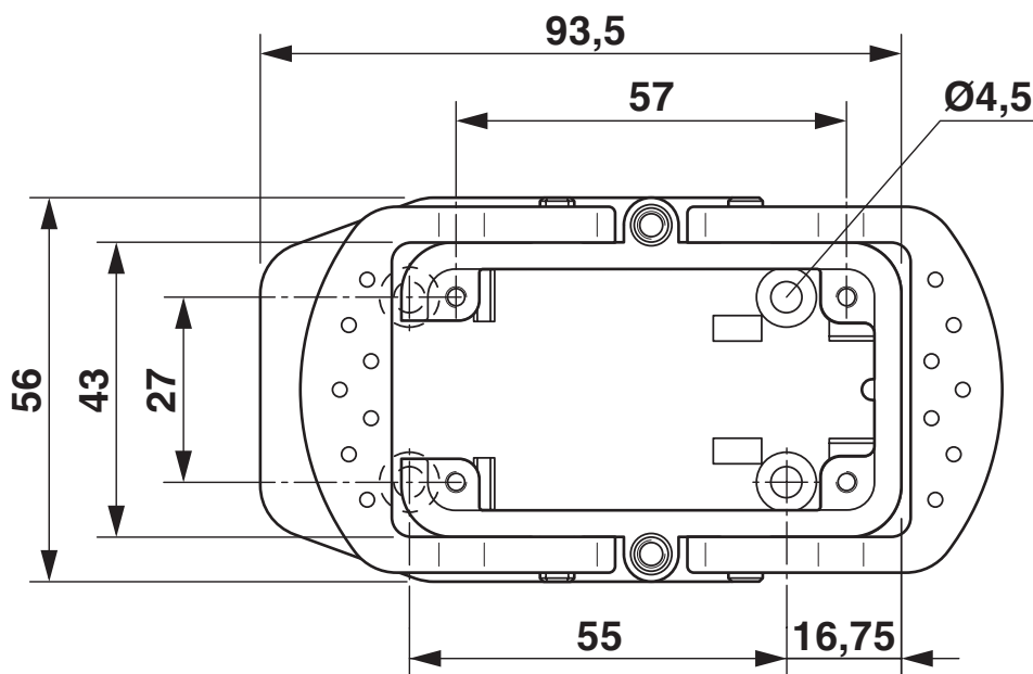
Esquema dimensiones vista desde arriba
