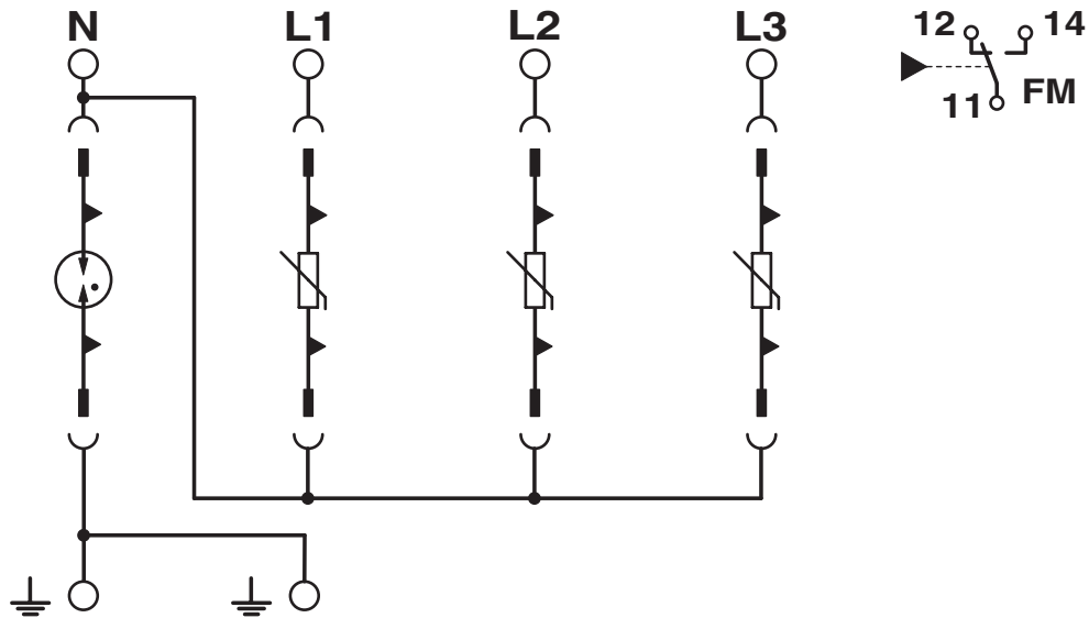
Schaltplan
