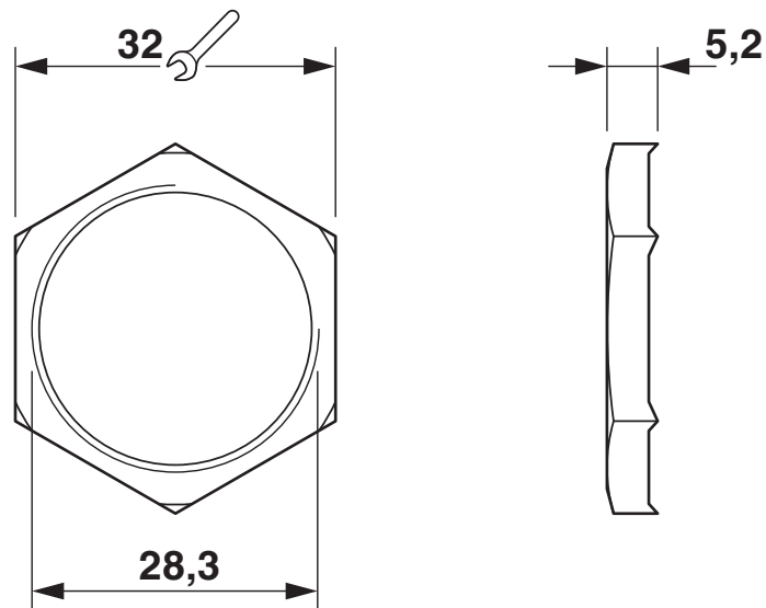
Maßzeichnung
