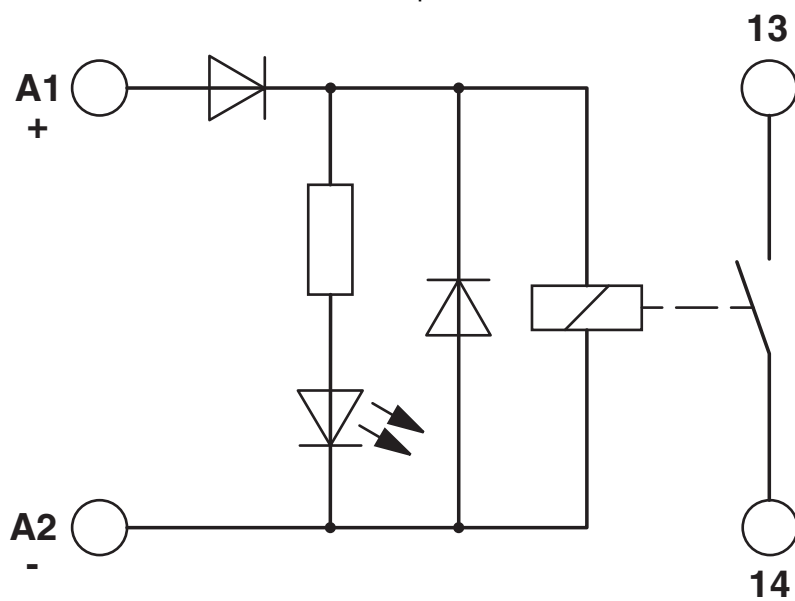
Schaltplan
