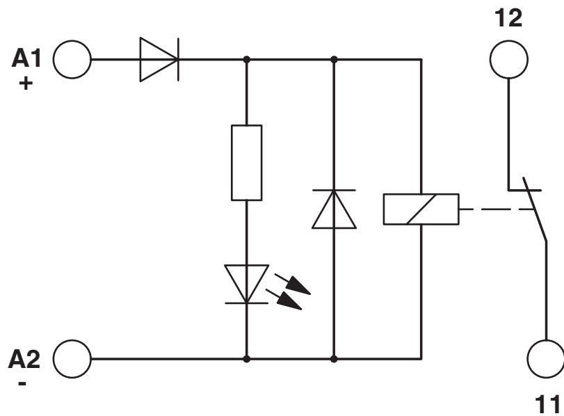
Schaltplan
