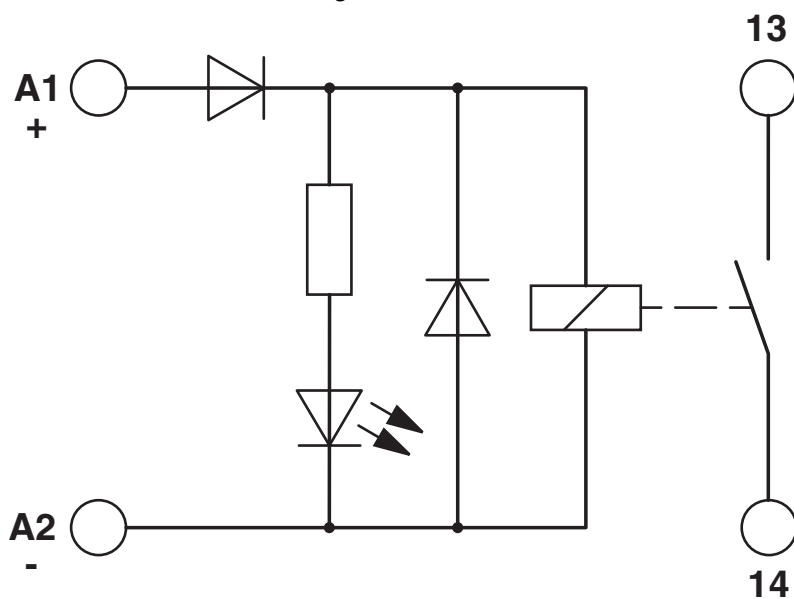
Diagrama eléctrico
