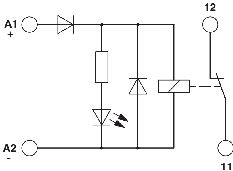
Diagrama eléctrico
