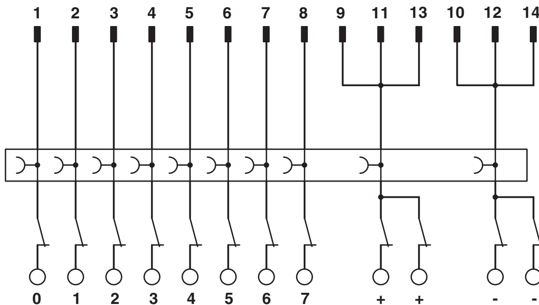
Schéma des connexions FLKM 14/KDS3-MT/PPA/PLC
