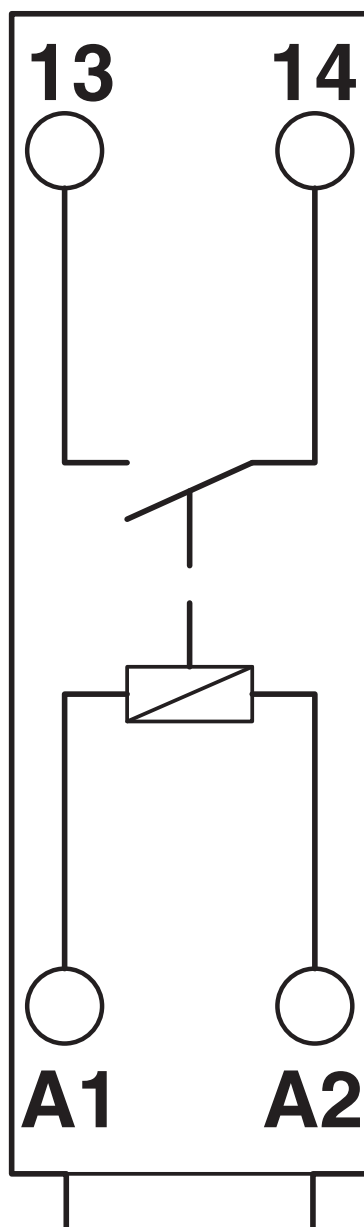
Diagrama eléctrico
