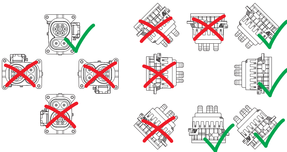
Anschlusszeichnung
