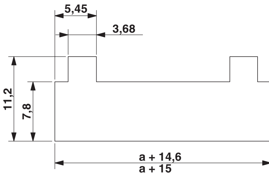
Plano esquemático
