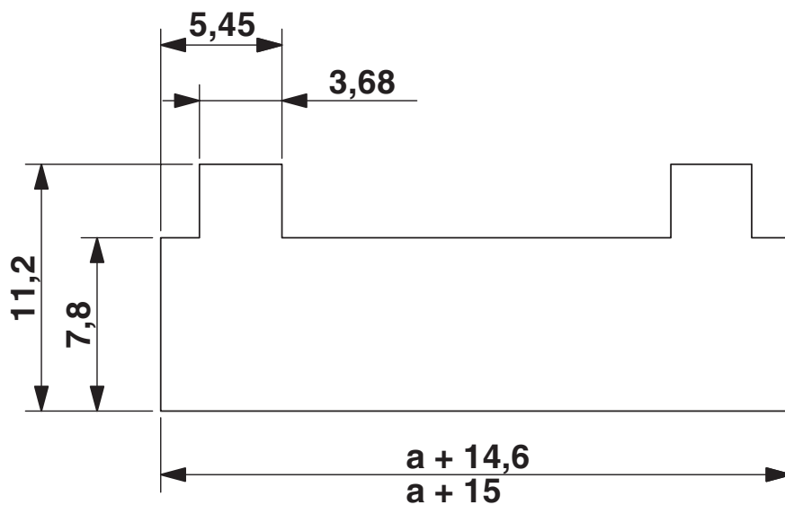
Dessin schématique
