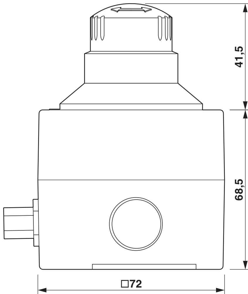
Maßzeichnung
