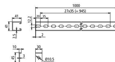
Maßbild MSC MDH V4A L1000 MZ V2A
