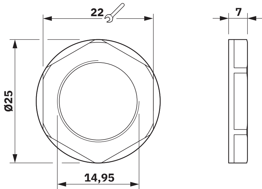
Maßzeichnung
