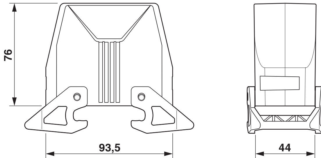
Maßzeichnung
