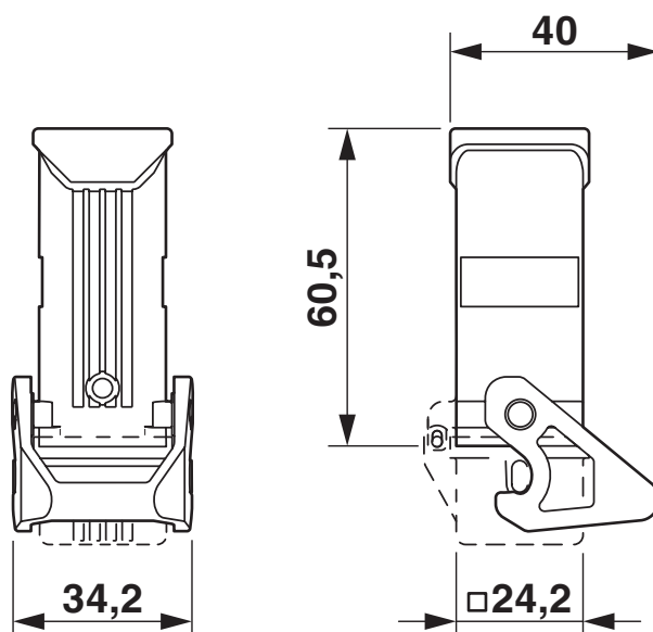
Dessin coté
