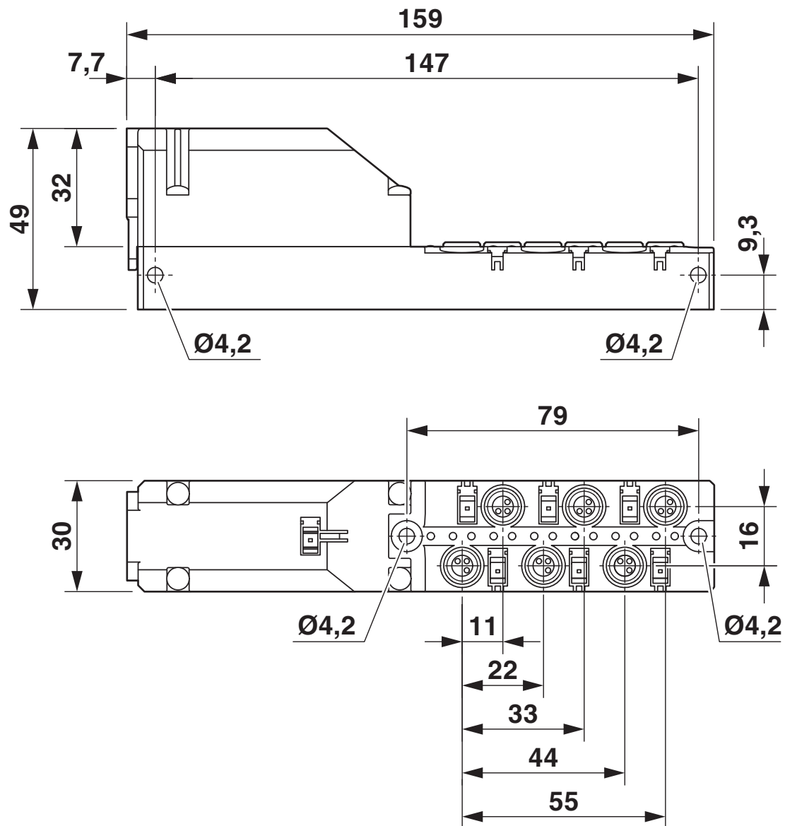
Maßzeichnung
