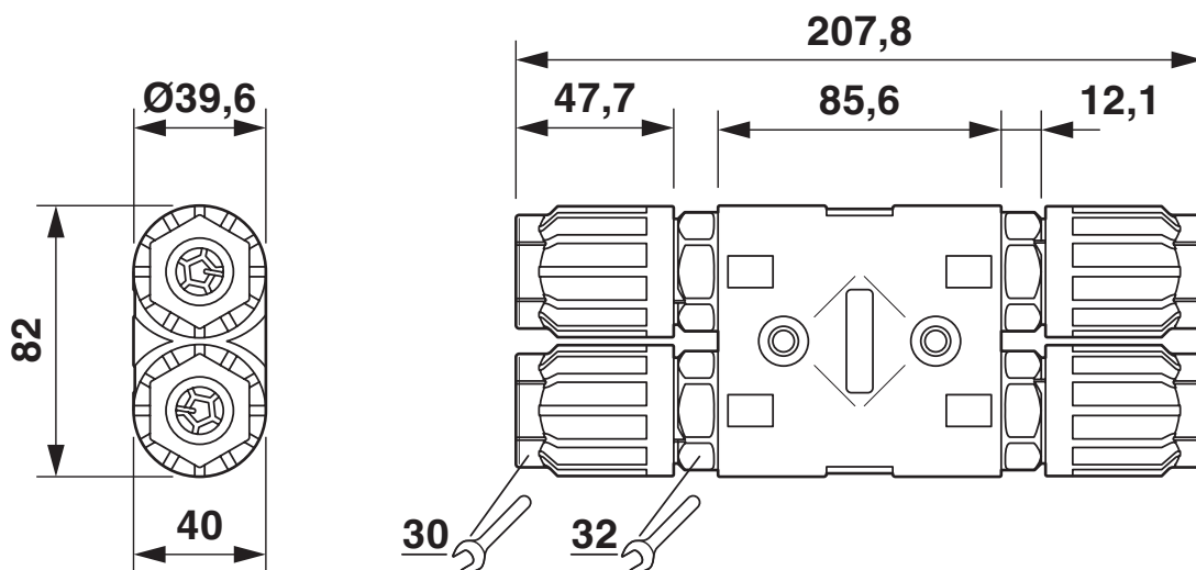
Maßzeichnung
