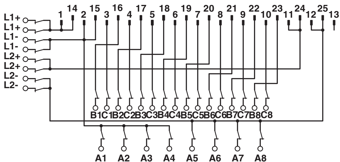
Esquema de conexiones FLKM-D25 SUB/B/KDS3-MT/TU810
