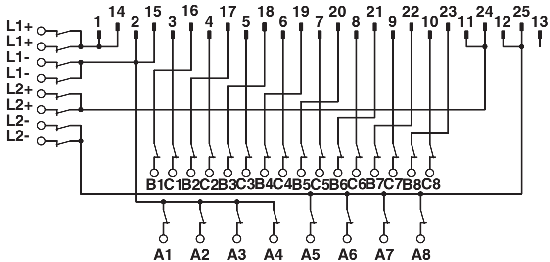
Schéma des connexions FLKM-D25 SUB/B/KDS3-MT/TU810
