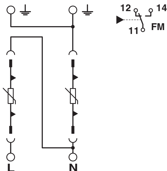
Diagrama eléctrico
