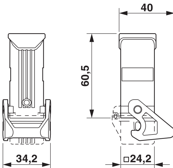
Maßzeichnung
