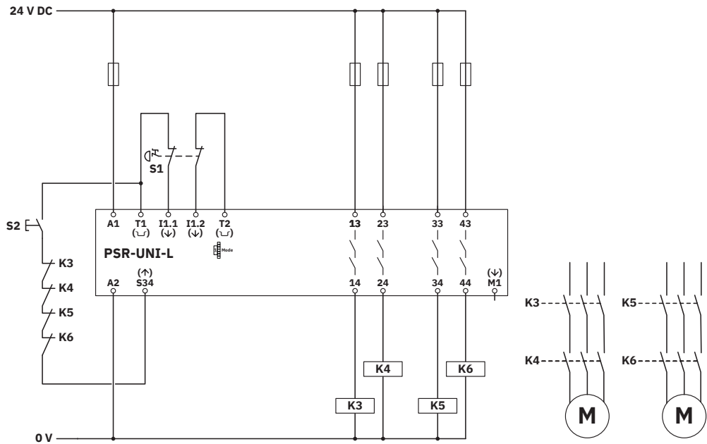
Diagrama eléctrico
