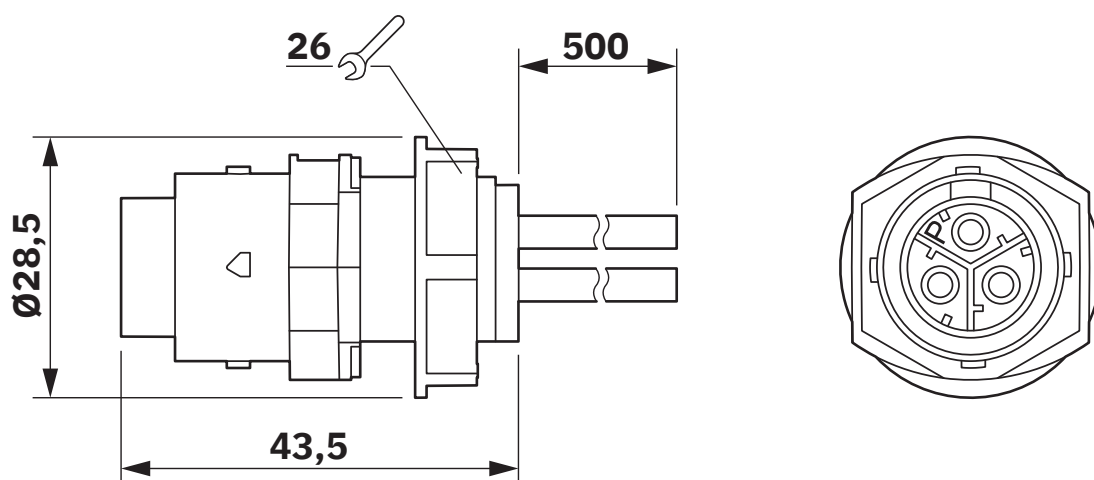
Maßzeichnung
