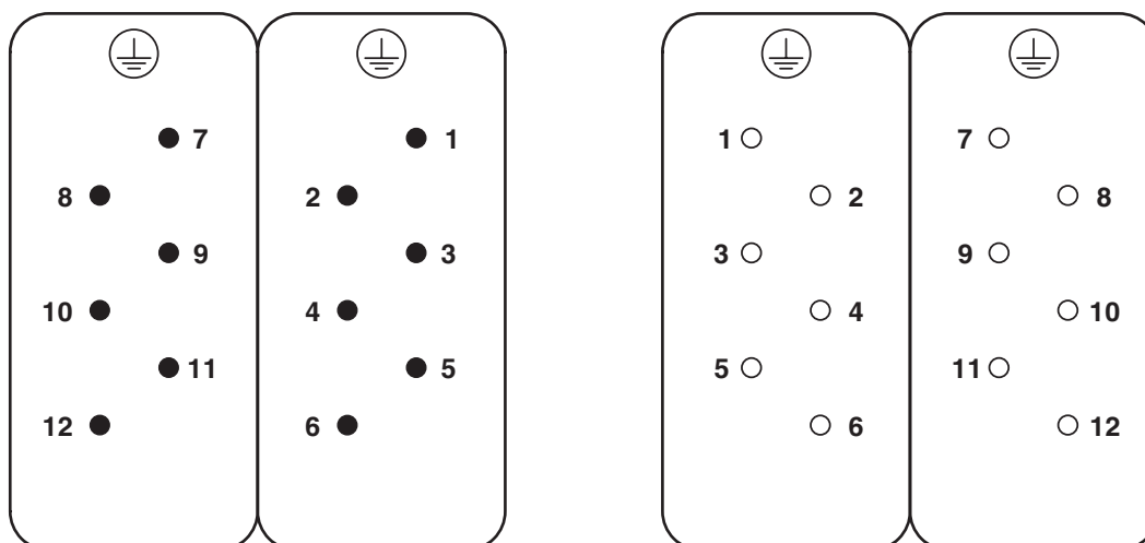
Esquema de polos Lado de conexión
