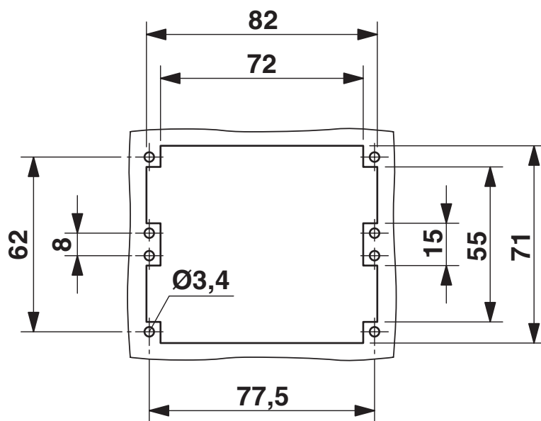
Dessin coté
