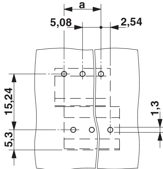
Bohrplan/Lötpadgeometrie
