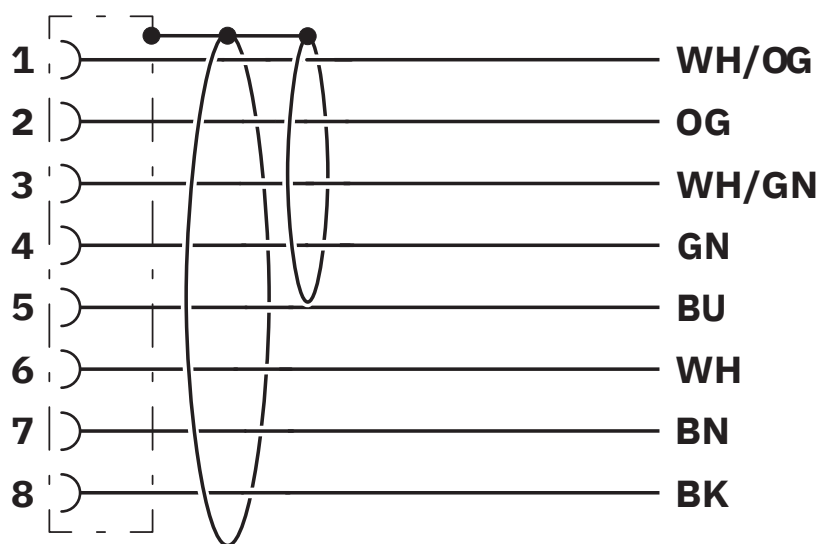
Diagrama eléctrico
