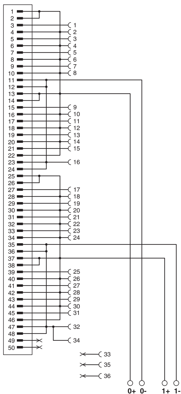
Diagrama eléctrico
