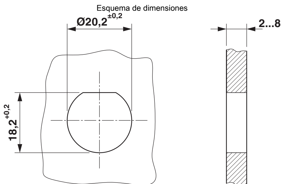
Dibujo acotado de QPD W 5 x 2,5 M20 sin tuerca
