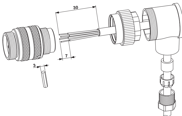
Funktionszeichnung
