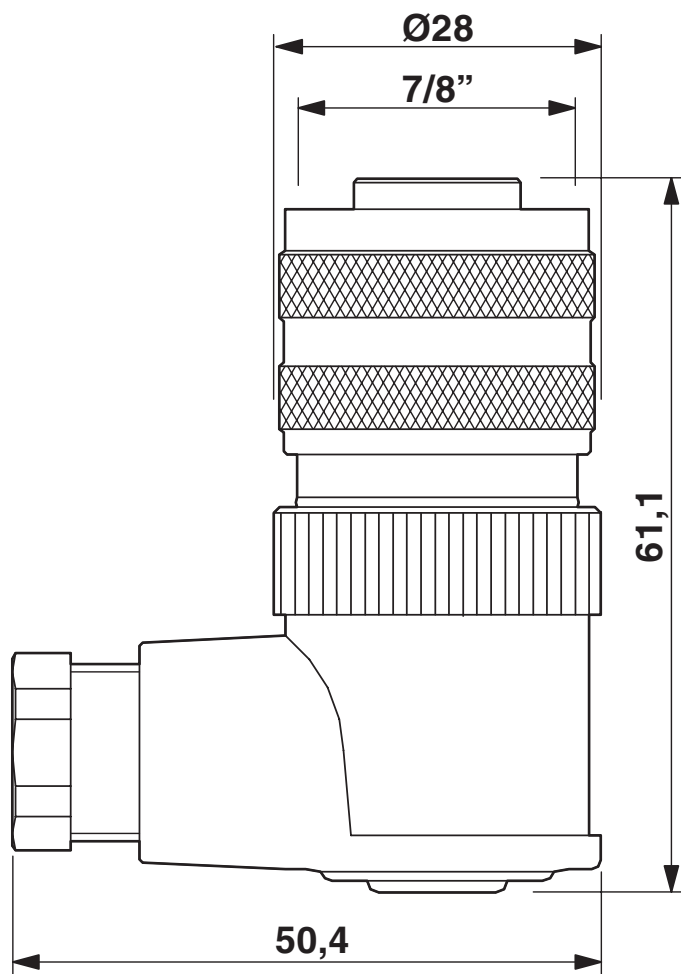
Maßzeichnung
