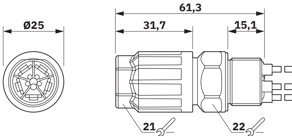
Maßzeichnung
