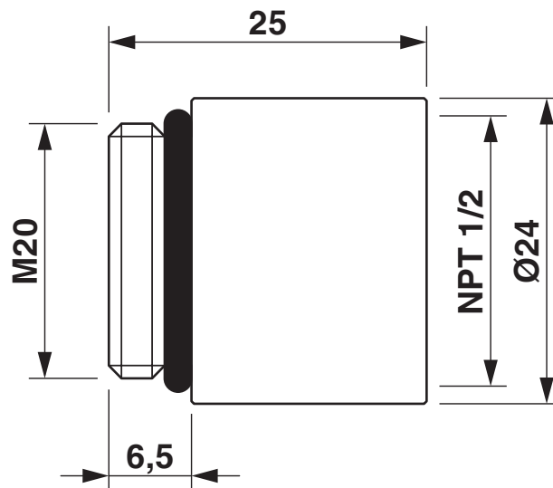
Maßzeichnung
