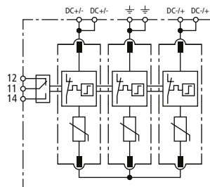
Prinzipschaltbild DG MD YPV 1500 FM
