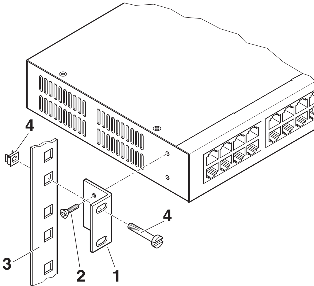
Applikationszeichnung
